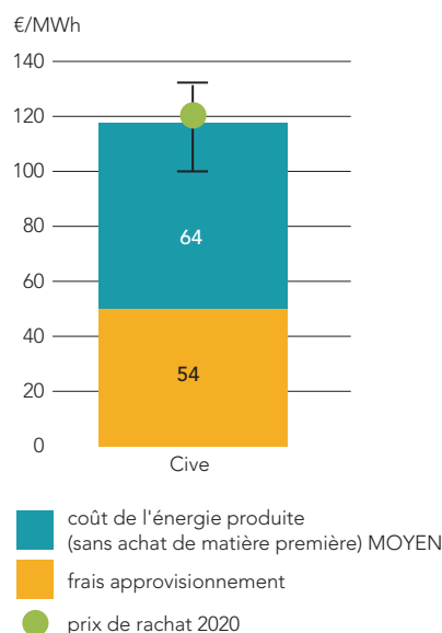
Figure 4 : Equilibre entre coût de production et prix de vente. Exemple de l'unité à injection 135 Nm 3 /h.
