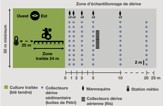
Figure 1 : Dispositif expérimental de mesure de dérive. Ce dispositif, utilisé en 2021, a été repris en 2022, mais une haie naturelle était présente entre 1,5 et 4 m, et deux distances de collecte ont été rajoutées à 15 et 25 m de la zone traitée. Sur ce schéma, le vent vient de l'Ouest et se dirige vers l'Est.
