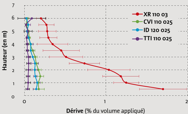
Figure 2 : Dérive sédimentaire (% du volume appliqué) à 1, 2, 3, 5, 10 et 20 m de la zone traitée (gauche) et dérive aérienne (% du volume appliqué) à 5 m de la zone traitée (droite), au stade DFE, pour les différents types de buses. Essai Arvalis Boigneville 31/05 & 01/06/2021.
